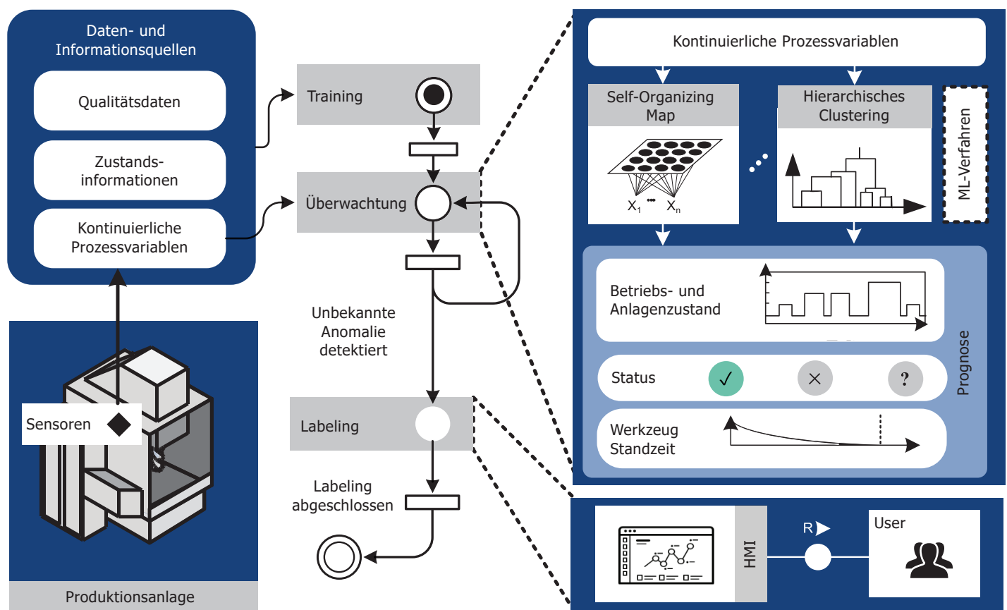
Abbildung 7: Ablauf und Architektur eines ML-basierten Prozessüberwachungssystems am Beispiel der spanenden Fertigung (in Anlehnung an [26])
