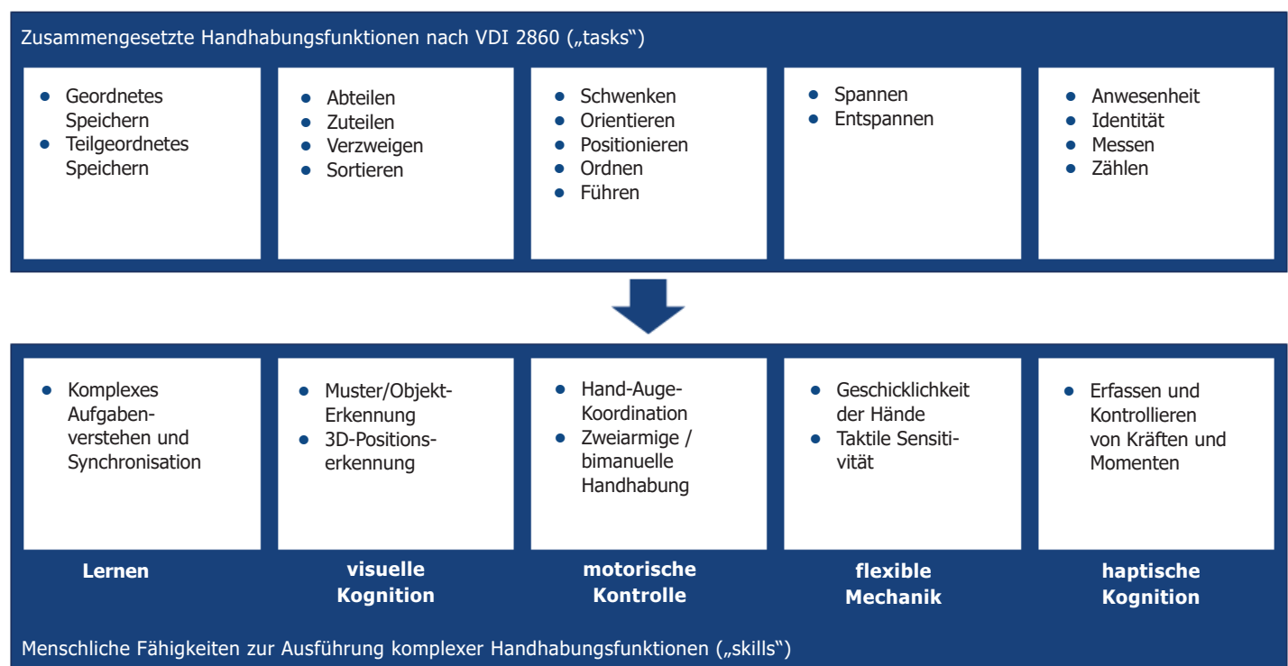
Abbildung 4: Systematische Abbildung von „tasks“ (produktionstechnische Kompetenz) und „skills“ (KI-Kompetenz) am Beispiel von Handhabungsfunktionen
