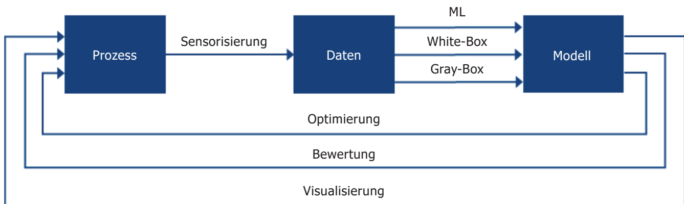
Abbildung 5: Produktionstechnisch prozessorientierter „Pull“-Ansatz zur Nutzung maschineller Lernverfahren in Anlehnung an [10]
